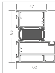
ościeżnica Termo ALU 68
