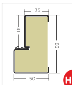
ościeżnica Termo ODS56
