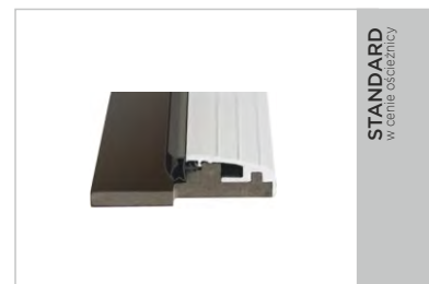
próg Termo ALU/PCV ODS68
