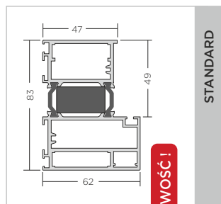
ościeżnica Termo ALU 68
