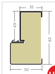
ościeżnica Termo ODS68
